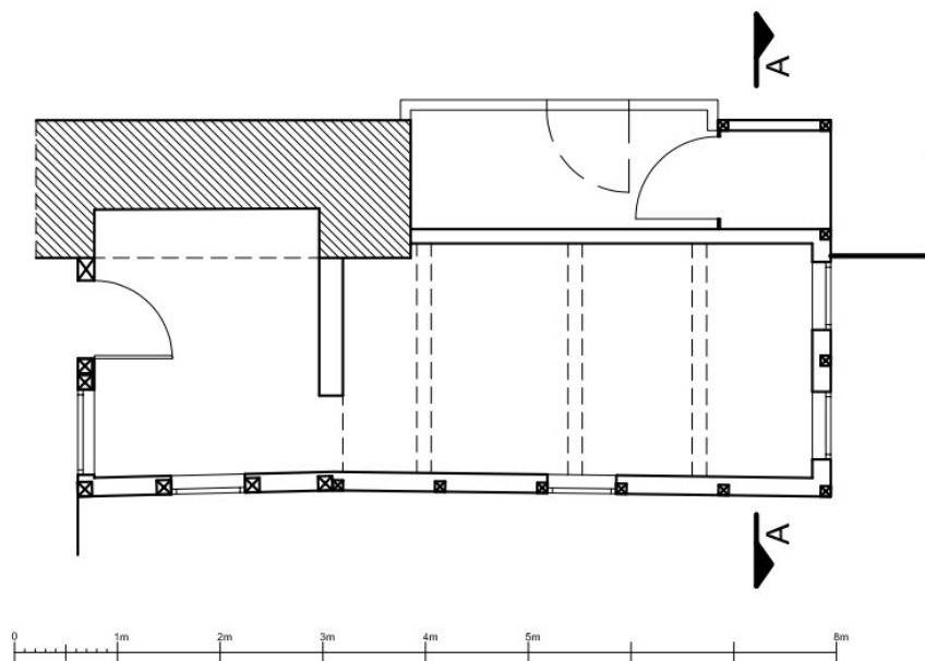
Rys.5 Rzut poziomy Wartowni
