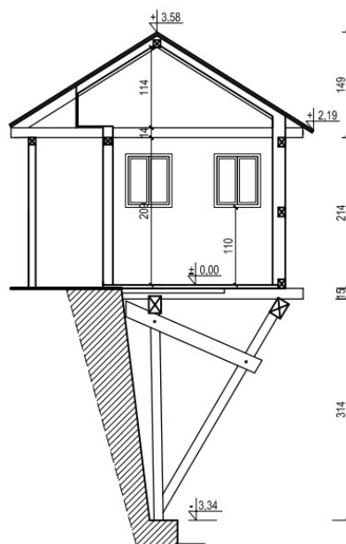
Rys.4 Przekrój przez Wartownie
