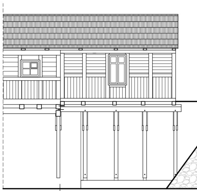
Rys. 6 Elewacja Południowa
